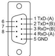
RS-422/RS-485-4w
