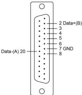
RS-485-2w
