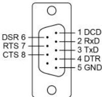
RS-232
