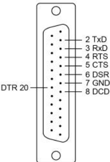
RS-232
