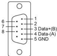
RS-485-2w
