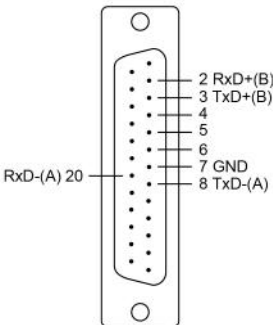
RS-422/RS-485-4w
